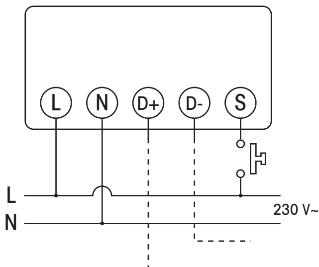
ESQUEMA DE CONEXIONES / CONNECTION DIAGRAM
