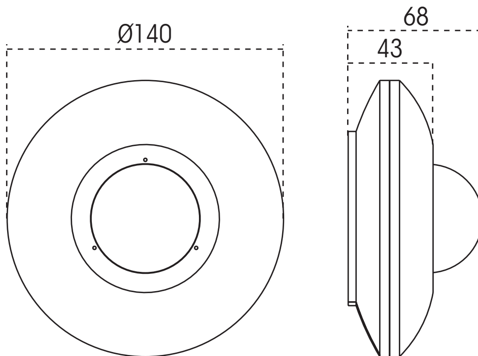
ESQUEMA DE DIMENSIONES / DIMENSIONS DIAGRAM
