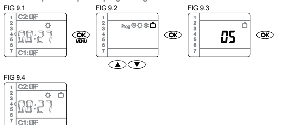
FIG. 9. Programar periodo de vacaciones de 5 días / 5 days holiday time programming
