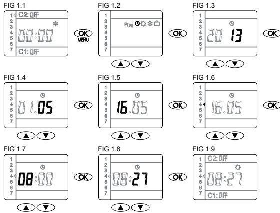
FIG. 1. Puesta en hora y fecha / Time and date setting
