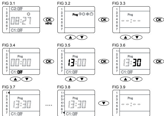
FIG. 3. Programar maniobra de apagado de lunes a viernes a las 13:30 en C1 / Switching OFF programing from Monday to Friday at 13:30 in C1
