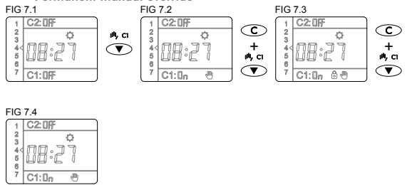
FIG. 7. Conmutación manual permanente / Permanent manual override
